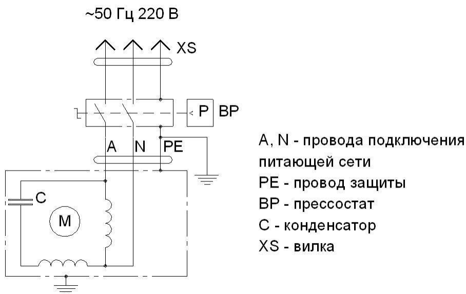
Рисунок А.1 - Схема электрическая принципиальная компрессоров СБ4/С-20.11047В, СБ4/С-24.11047В, СБ4/С-50.11047В, СБ4/С-20.11048В, СБ4/С-24.11048В, СБ4/С-50.11048В
