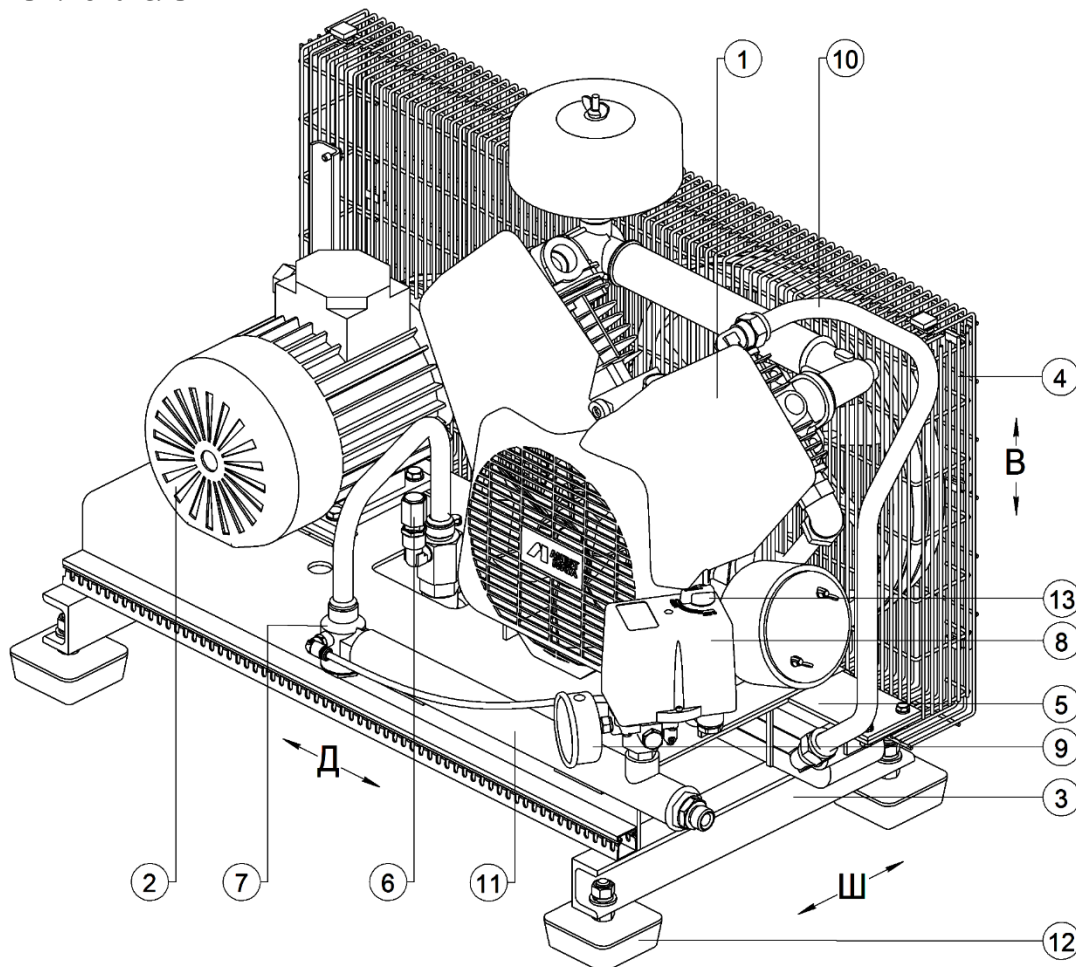
Рисунок 4 - Общий вид компрессора СБ4-F22
