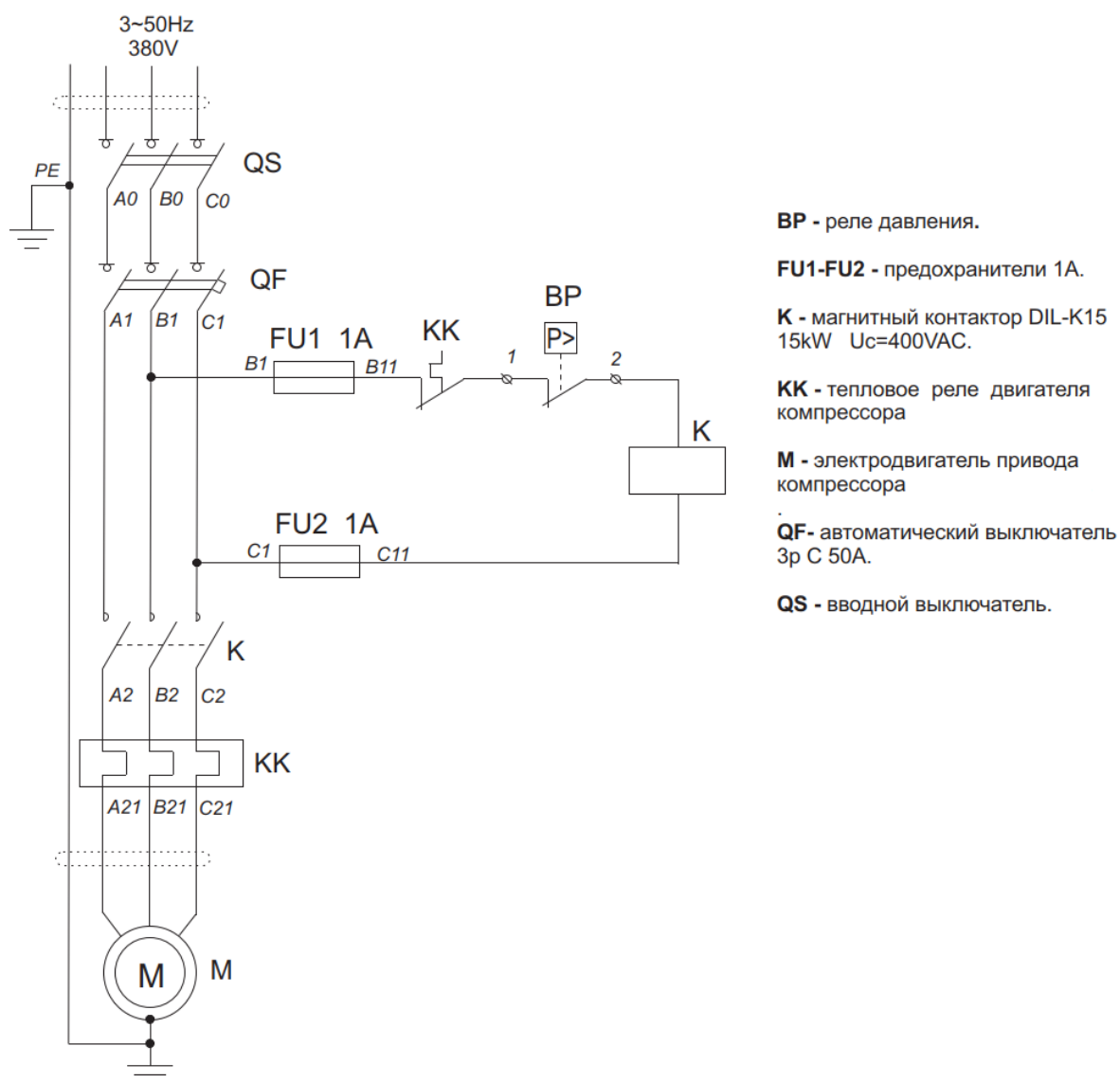
Рисунок А.1 - Схема электрическая принципиальная компрессоров СБ4-500.F55, СБ4-500.F55, СБ4-500.F55/14
